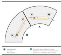
Detalle bajo tablero de la conexión eléctrica entre mesas. Detail of the electrical connection between tables under the work top. Détail sous plateau de raccordement électrique entre tables.
